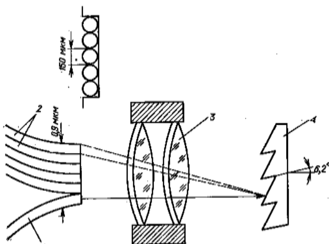
Рис. Л.4.1. Устройство пятиканального демультиплексора:
